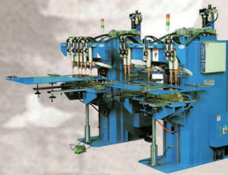
멀티 스포트 용접기 MULTI SPOT WELDER
